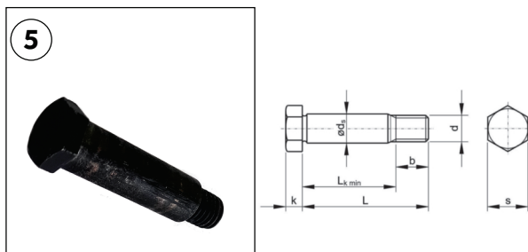
PARAFUSO SEXTAVADO DIN 610 M8X40 – ROSCA CURTA
